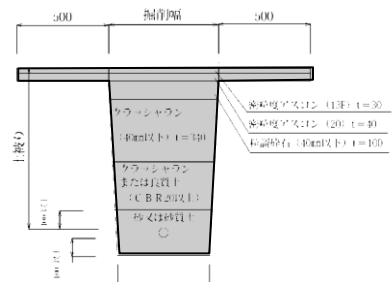
本復旧標準断面図 S=1 : 50
