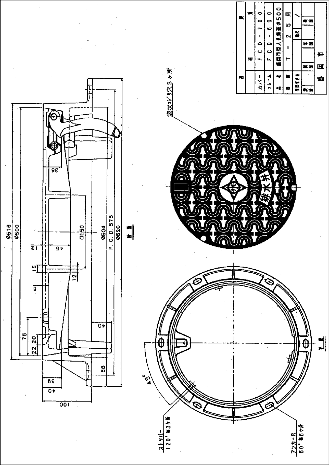
別図 3 - 1 「鉄蓋標準図 (T-25用)」
