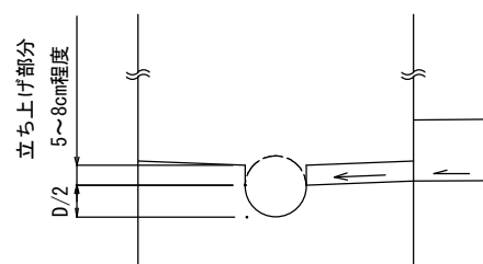
B-B' 断面
