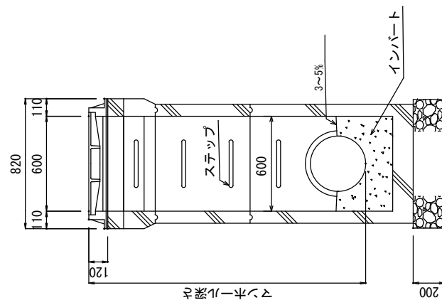
横断面図
