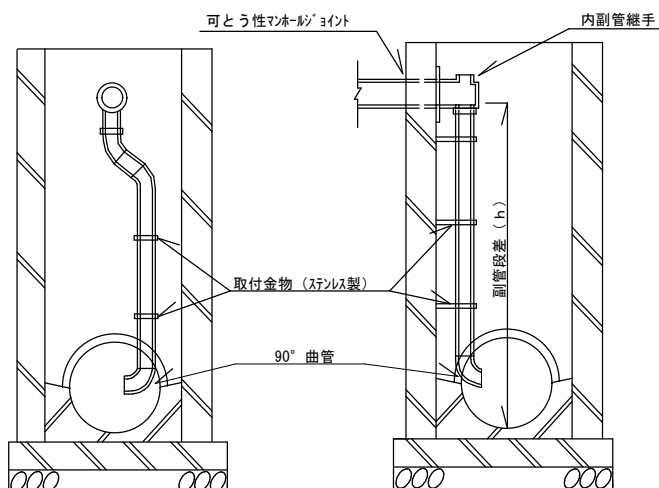
断面図
