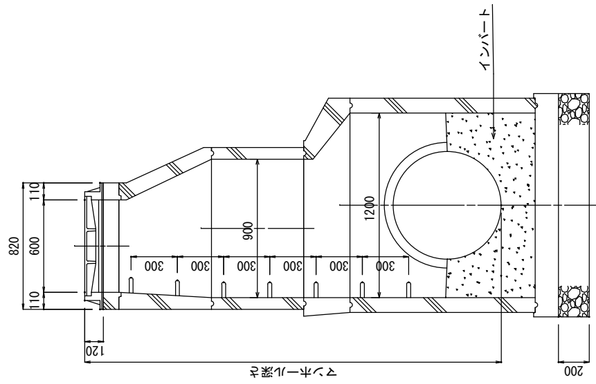
横断面図
