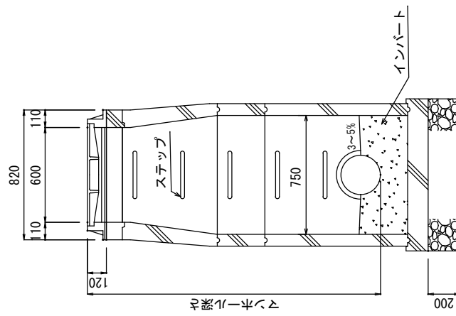
横断面図
