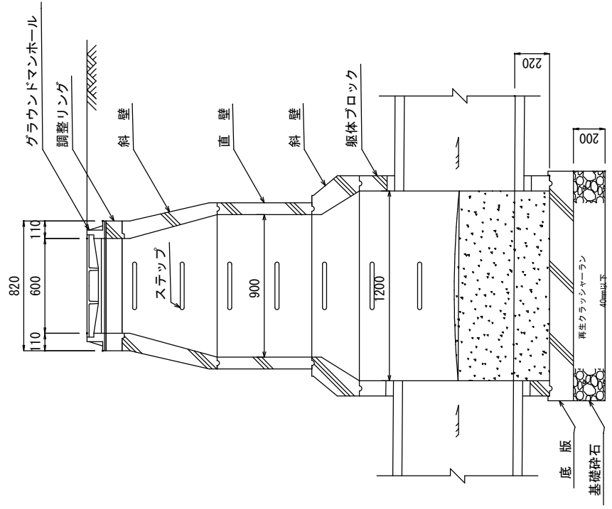
縦断面図
