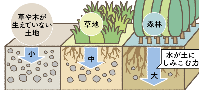
植生による雨水の浸透能の違い
